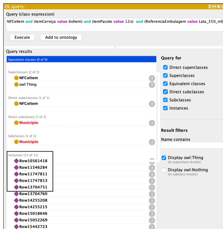
Figura 3 – Resultado da DL Query com a seleção de 11 instâncias de sentença completas da NFC- e . Detalhe para as 5 primeiras linhas. Fonte: Dados da pesquisa, 2024.
